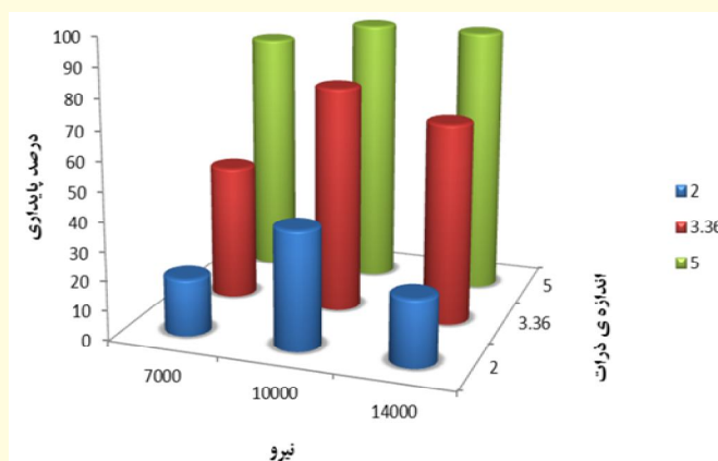
شکل ۳- اثر اندازه‌ی ذرات بر پایداری پلت در نیروهای مختلف و رطوبت ۶ درصد
